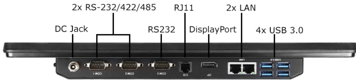
Bottom
